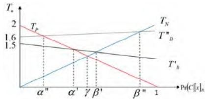
图 14 分段延迟代价敏感三支决策模型 4 示意图
