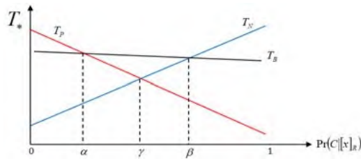
图 4 二支决策情况下, T_N 、 T_P 、 T_B 之间的拓扑关系示意图
